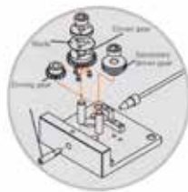
The structure of solder wire cutting system Diagramma sistema di taglio filo
